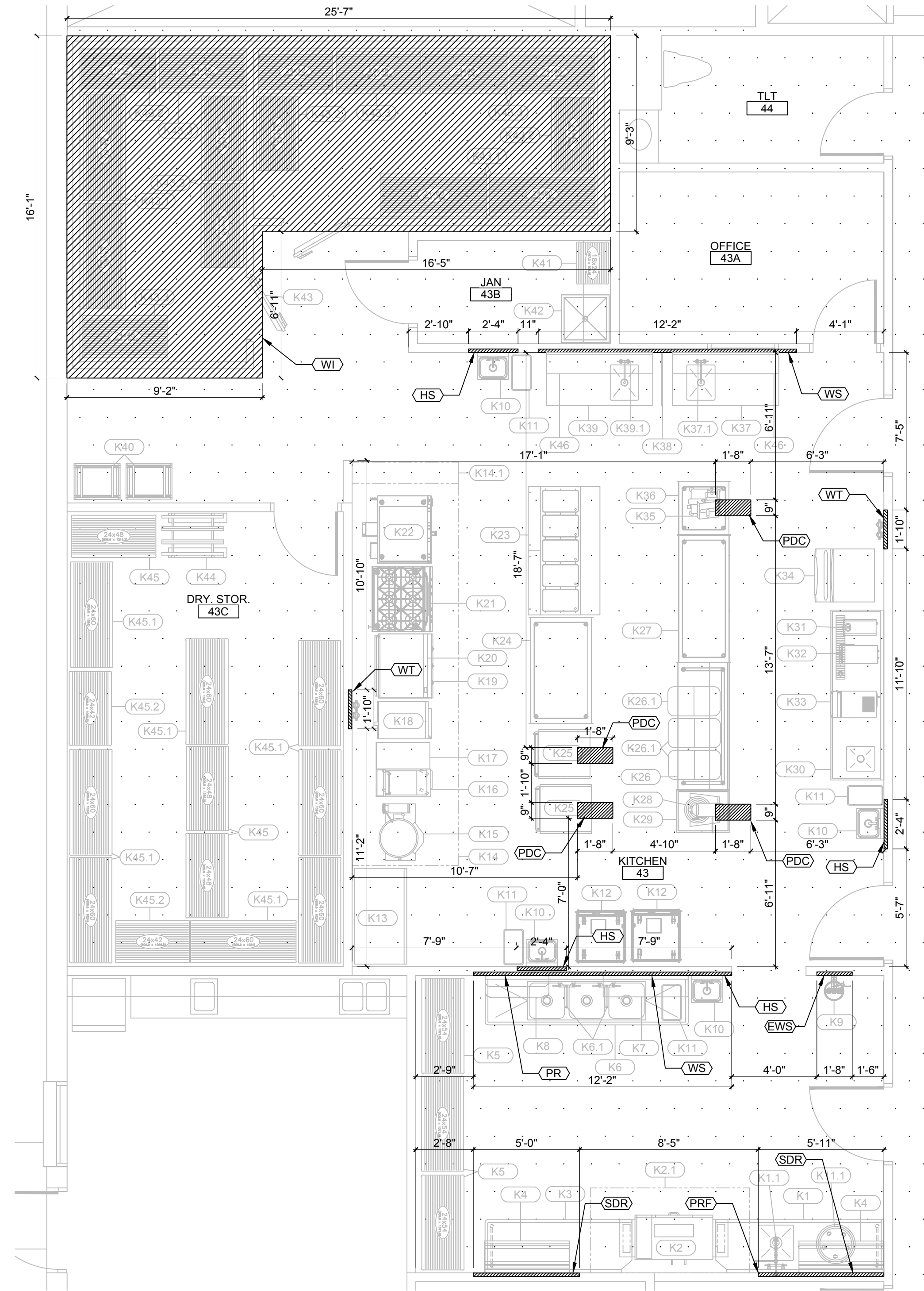
PLAN TRUE 1 SCALE: 1/4" = 1'-0"
