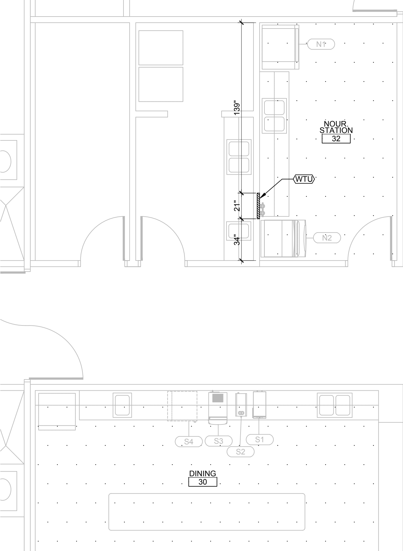
PLAN TRUE 2 SCALE: 1/4" = 1'-0"
