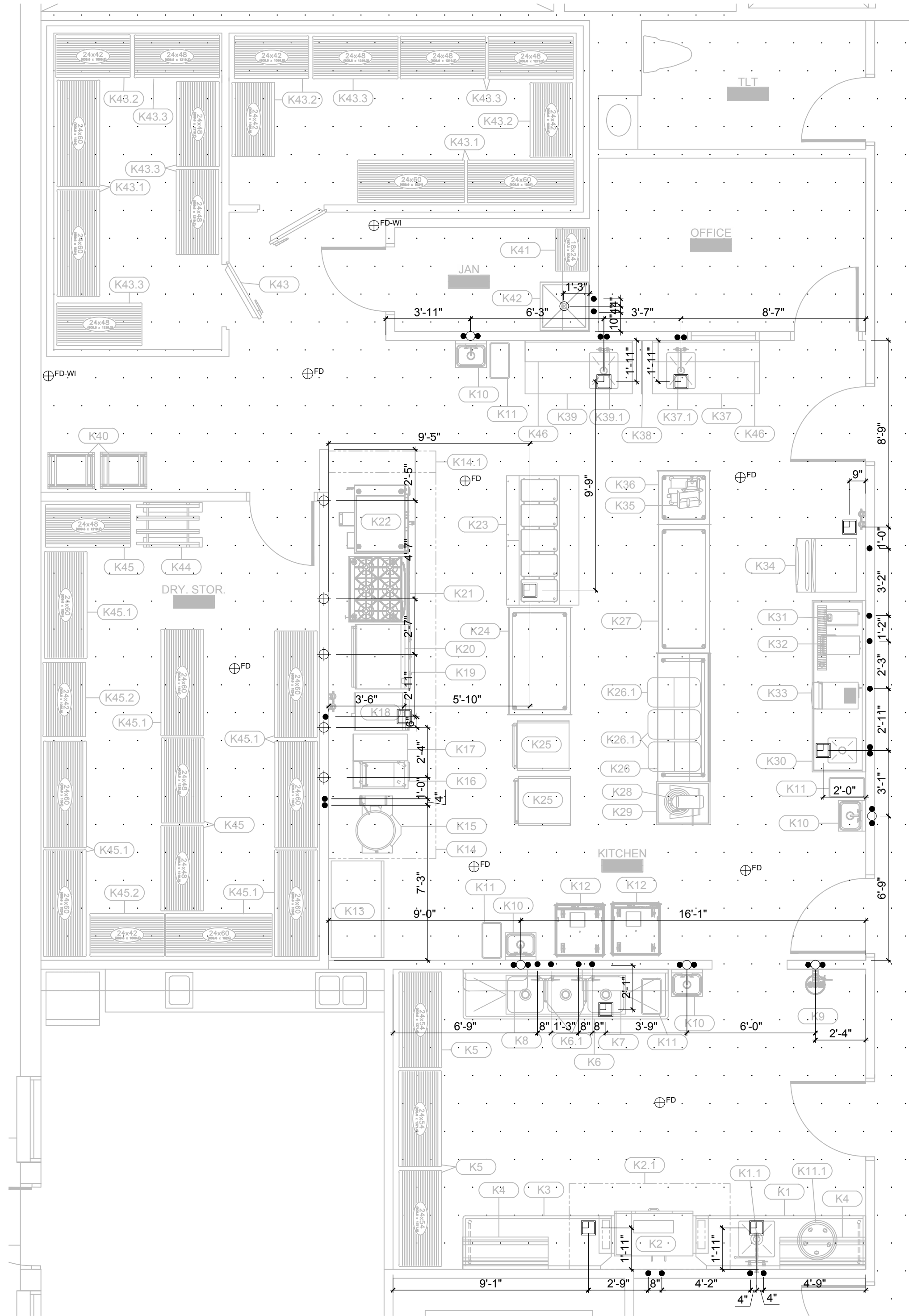
PLAN TRUE 1 SCALE: 1/4" = 1'-0"
