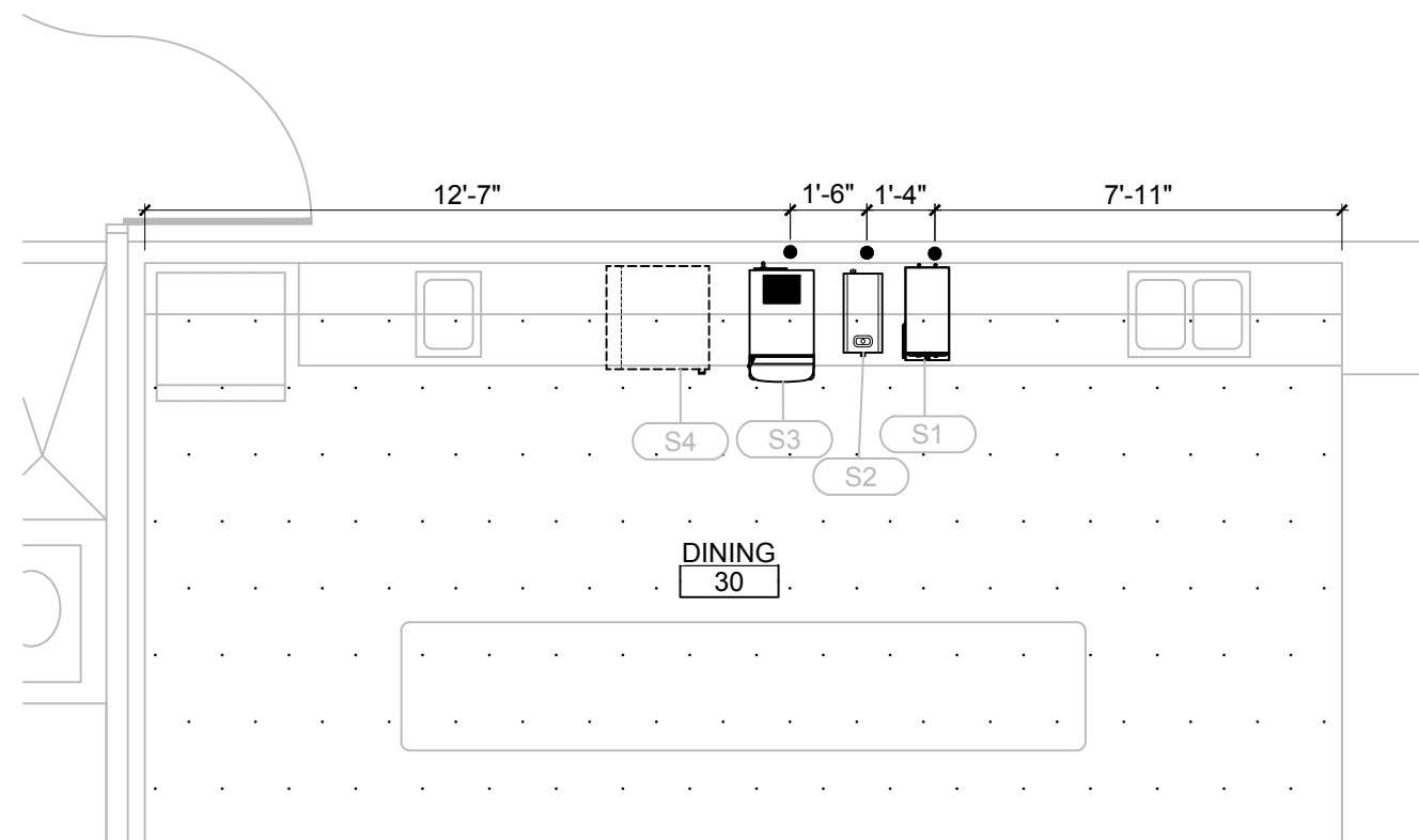
PLAN TRUE 2 SCALE: 1/4" = 1'-0"
