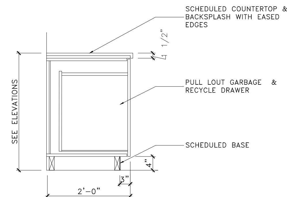
Base Cabinet - Garbage SCALE: \frac{3}{4}" = 1'-0"
